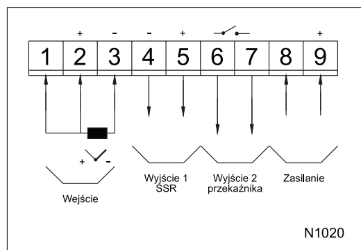
Schemat połączeń
