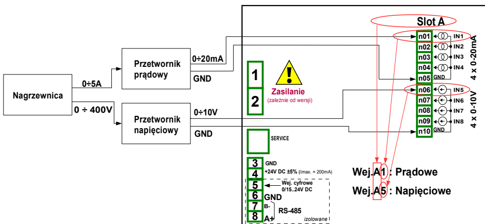
Rys. 7.61. Schemat połączeniowy dla modułu UI4
