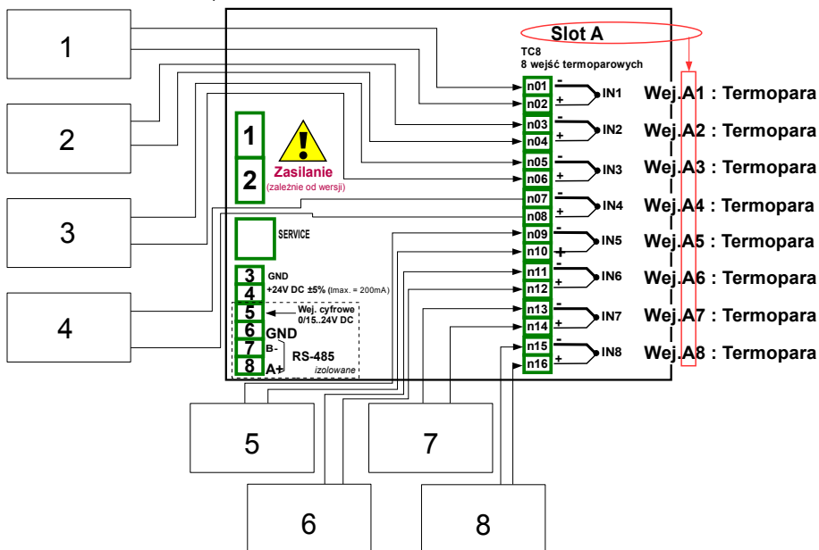
Rys. 7.74. Schemat połączeniowy dla modułu TC8
