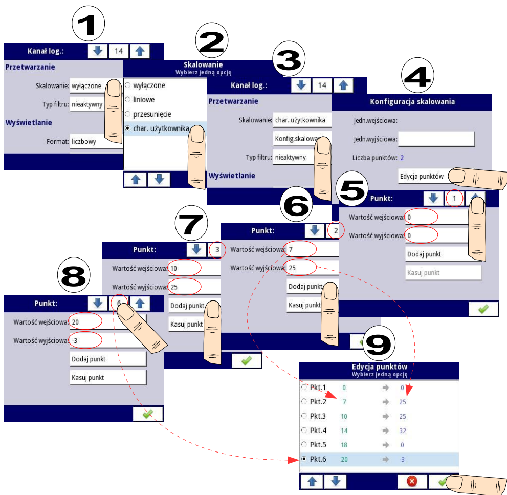
Rys. 7.39 Sposób konfiguracji przykładowej charakterystyki użytkownika
