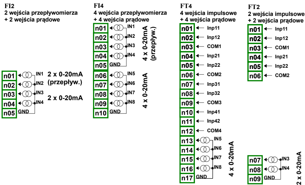
Rys. 4.13. Moduły do pomiaru przepływu
