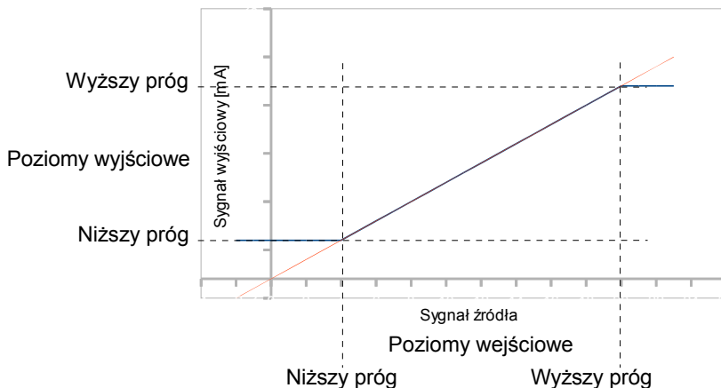
Rys. 7.101. Równanie transmisji (liniowe) sygnałów wejście - wyjście
