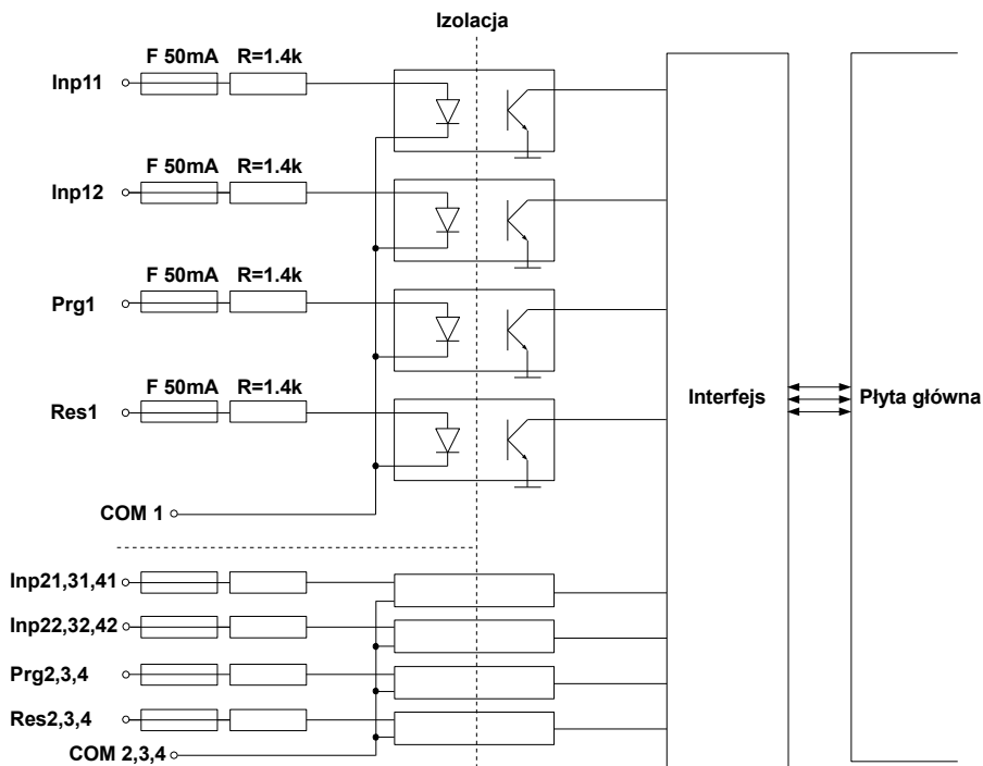
Rys. 8.20. Struktura wewnętrzna optoizolowanego modułu liczników uniwersalnych
