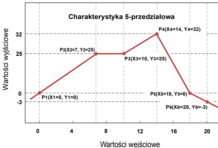
Rys. 7.38 Przykładowa charakterystyka użytkownika
