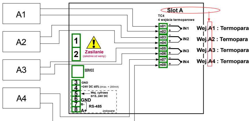
Rys. 7.67 Schemat połączeniowy dla modułu TC4
