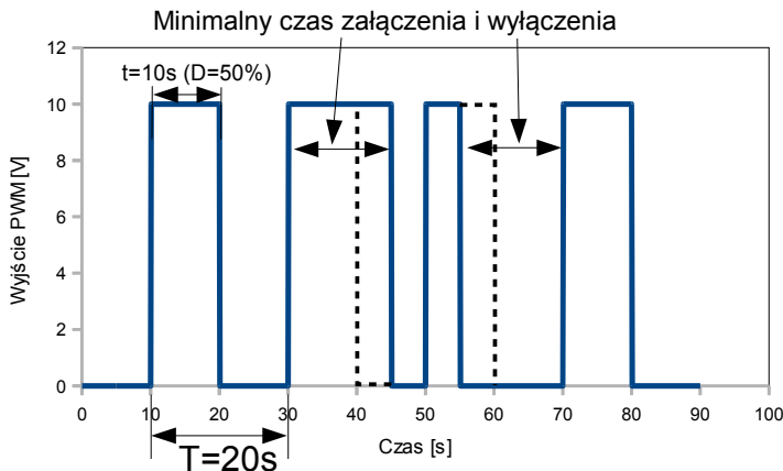
Rys. 7.92. Przykładowy przebieg wyjściowy przełącznika SSR w trybie PWM
