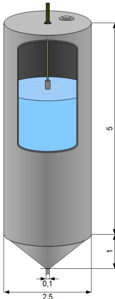
Rys. 7.22 Przykładowy zbiornik w kształcie połączonego walca i stożka
