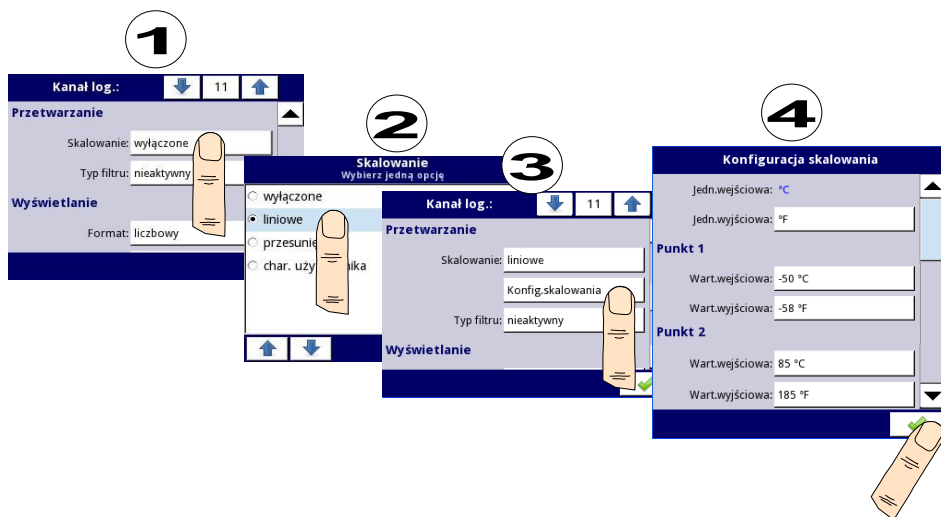
Rys. 7.37. Przykładowa konfiguracja bloku parametrów Przetwarzanie
