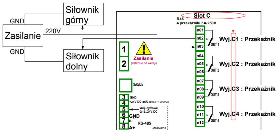
Rys. 7.71. Schemat połączeniowy dla modułu R45
