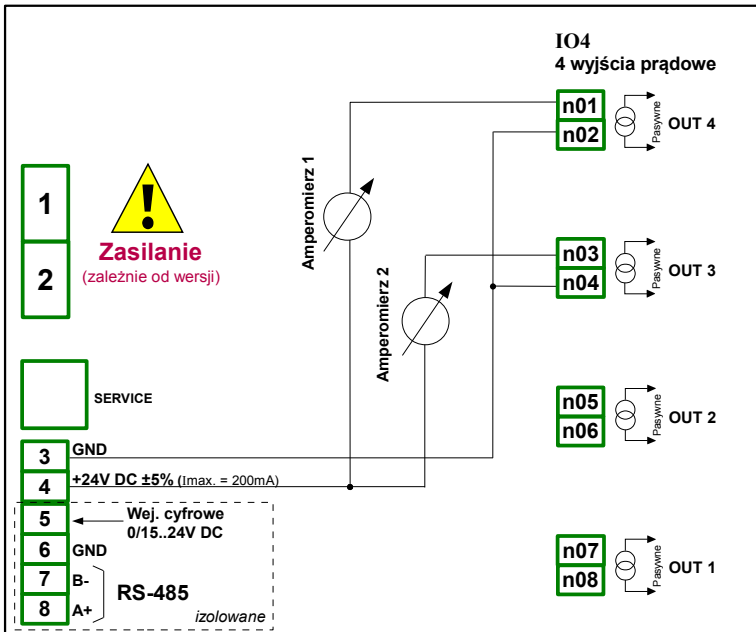
Rys. 8.30. Podłączenia dla Pasywnego wyjścia prądowego od strony GND
