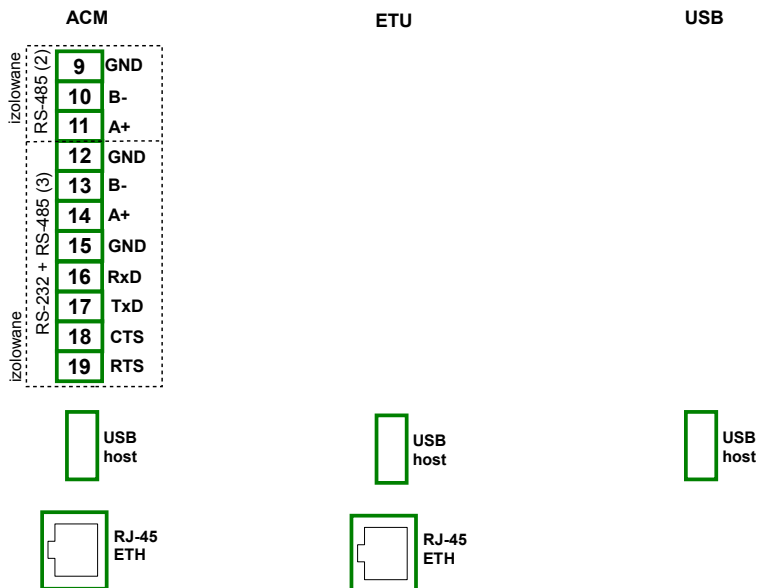
Rys. 8.33. Moduły komunikacyjne: ACM, ETU oraz USB (tylne - tylko USB host)
