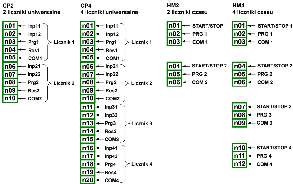
Rys. 4.18. Moduły liczników uniwersalnych oraz liczników czasu
