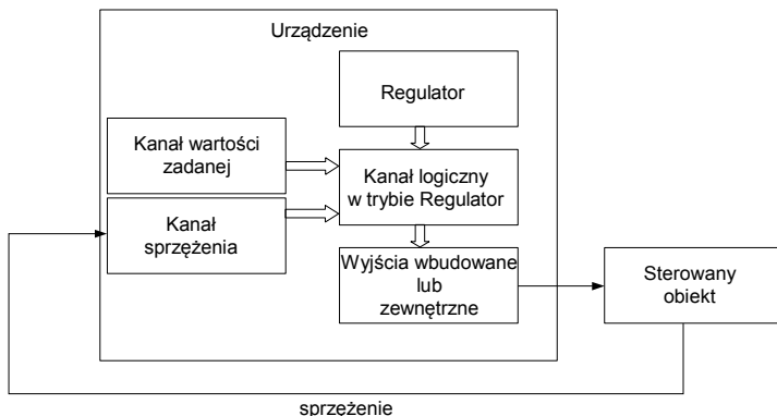
Rys. 7.114. Schemat blokowy procesu sterowania obiektem przy wykorzystaniu regulatorów
