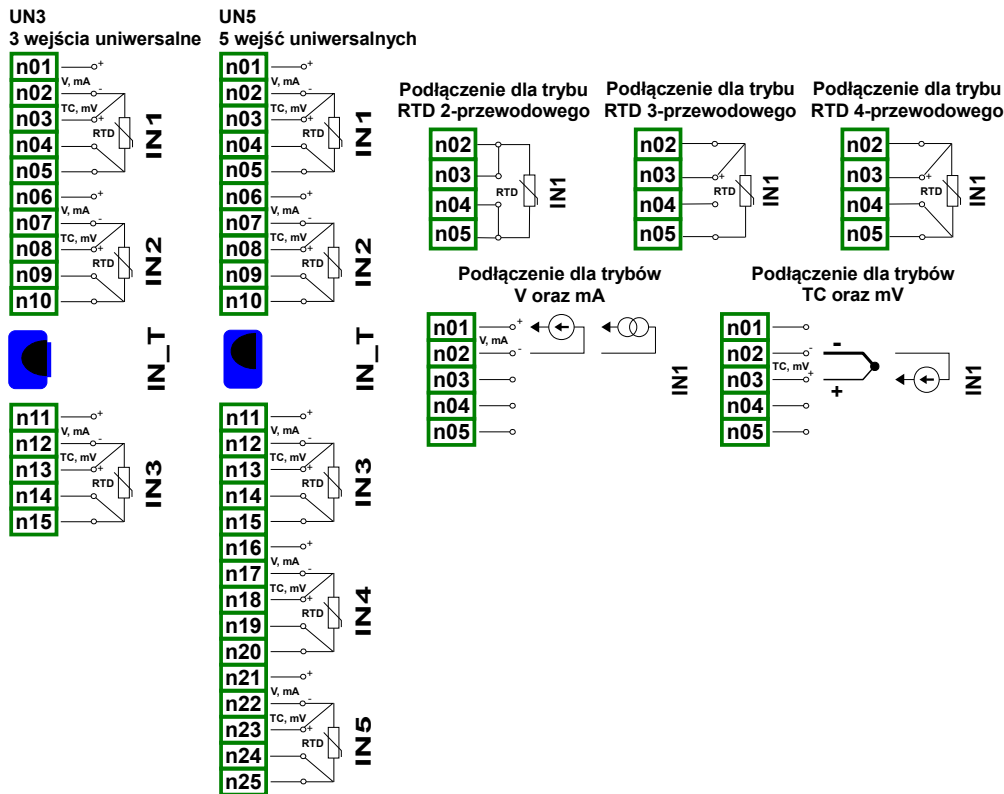
Rys. 8.15. Moduły wejść uniwersalnych
