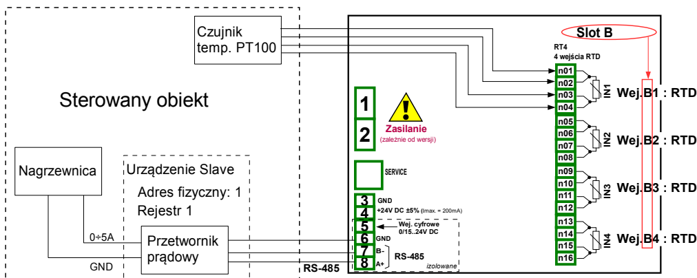
Rys. 7.76. Schemat połączeniowy dla modułu RT4 i portu Modbus MB1
