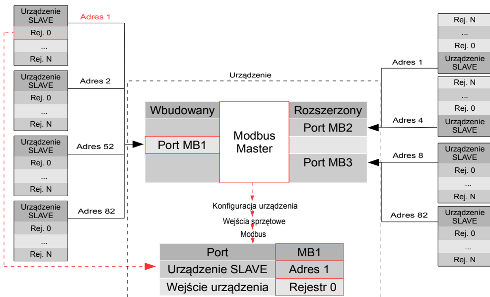
Rys. 7.52. Przykładowy schemat blokowy konfiguracji protokołu Modbus zaimplementowanego w urządzeniu
