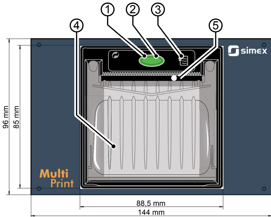
Rys. 8.34. Widok płyty czołowej
