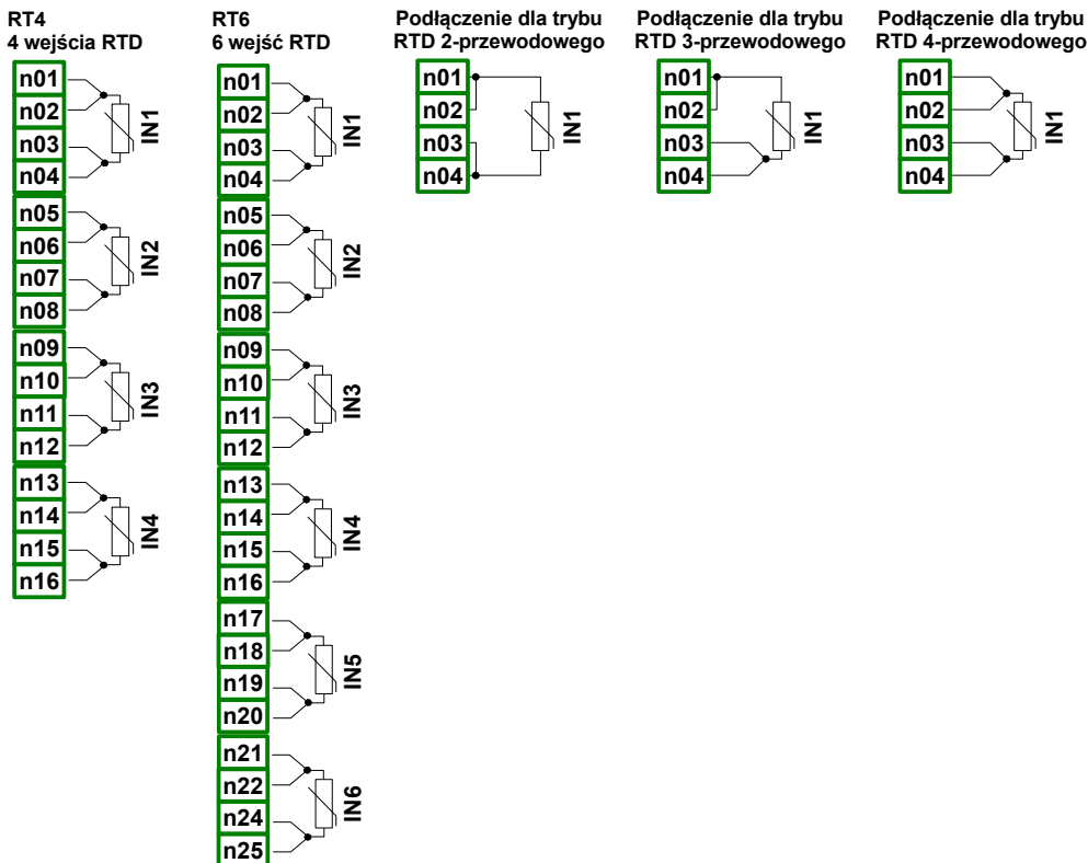
Rys. 8.14. Moduły RTD
