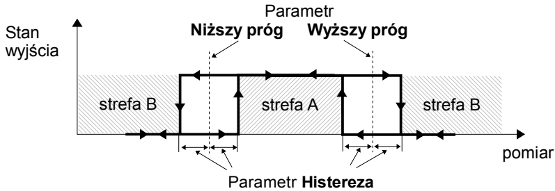
Rys. 7.86. Sterowanie dwuprogowe wyjścia przekąźnikowego
