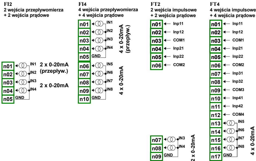
Rys. 8.10. Moduły przepływowierzowe
