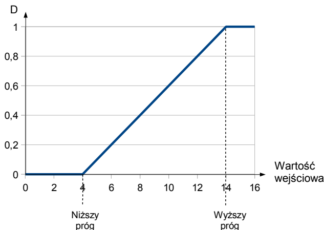
Rys. 7.91. Charakterystyka wejściowo - wyjściowa sygnału w trybie PWM dla parametrów: Niższy próg=4, Wyższy próg=14
