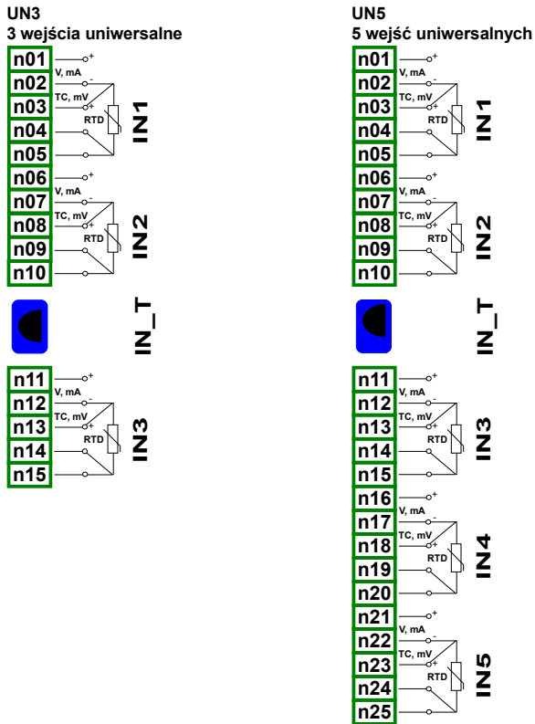
Rys. 4.16. Moduły wejść uniwersalnych
