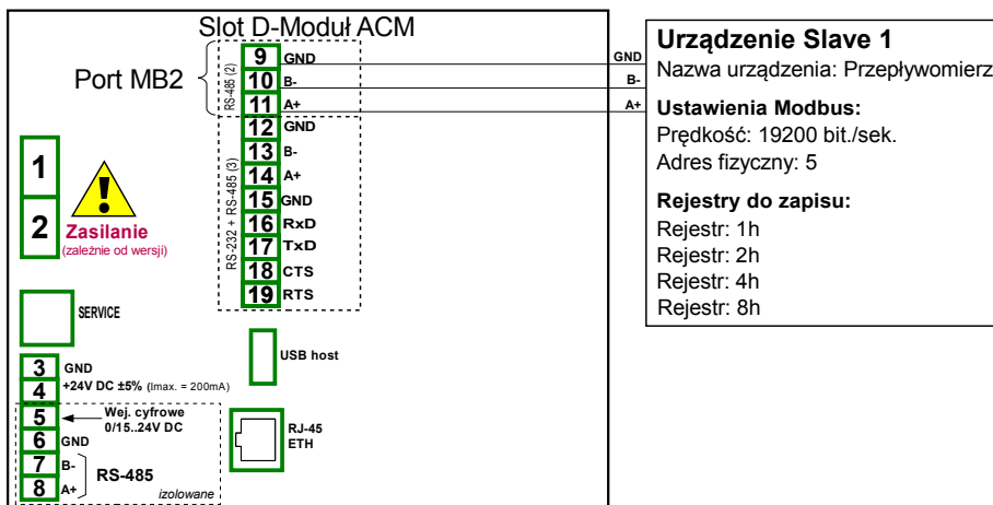
Rys. 7.102. Schemat połączeniowy dla portu Modbus MB2
