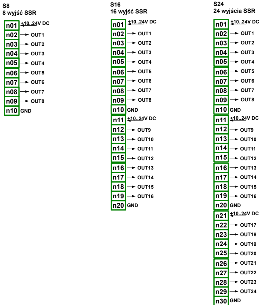
Rys. 4.19. Moduły wyjść typu SSR
