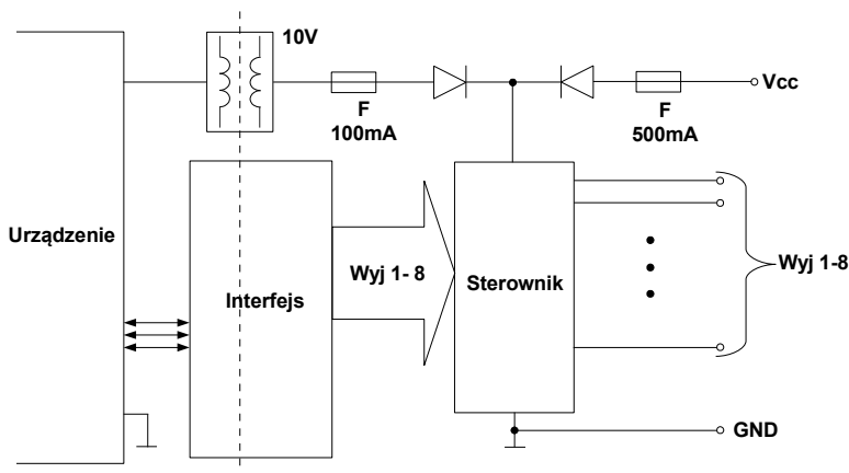
Rys. 8.24. Struktura wewnętrzna modułu wyjściowego SSR (8 wyjść)
