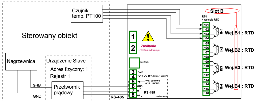
Rys. 7.116. Schemat połączeniowy dla modułu RT4 i portu Modbus MB1
