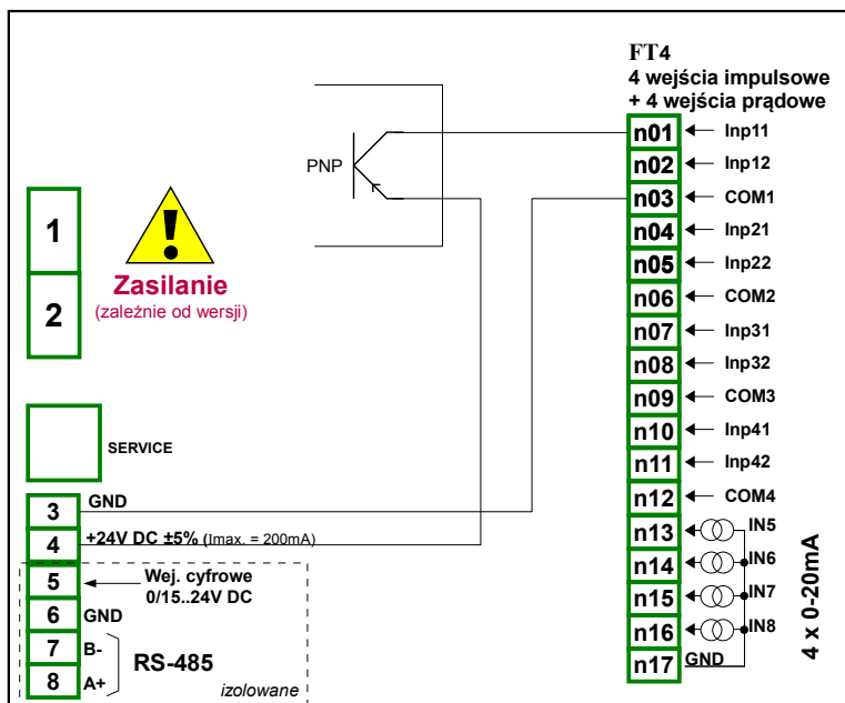
Rys. 8.11. Schemat połączeniowy dla modułu FT4 i czujnika typu PNP
