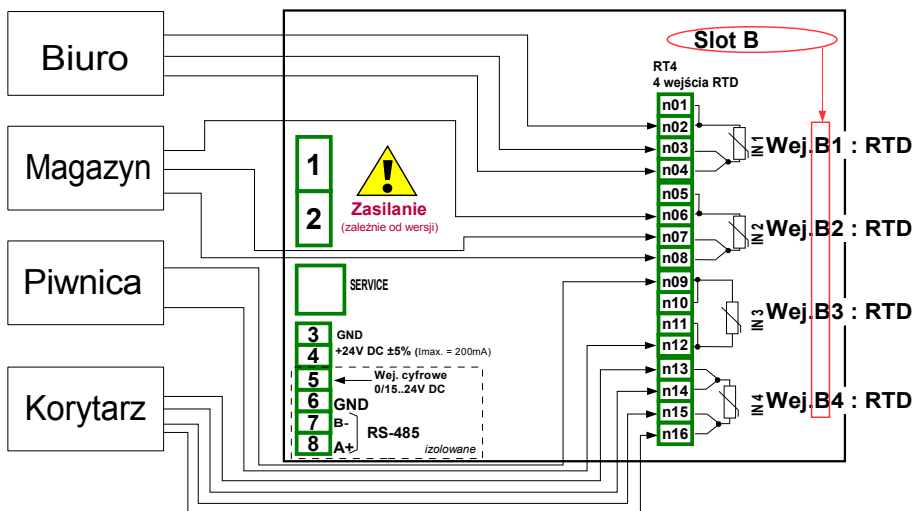
Rys. 7.69. Schemat połączeniowy dla modułu RT4
