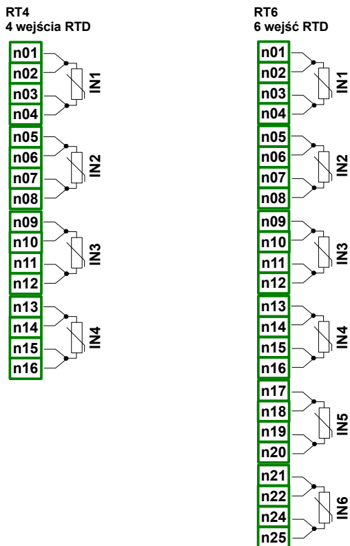
Rys. 4.15. Moduły wejść RTD
