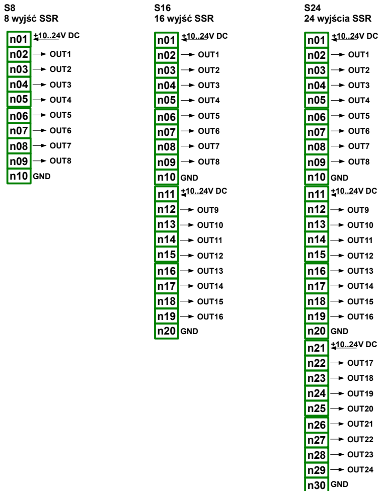
Rys. 8.23. Moduły wyjść przekaźnikowych typu SSR
