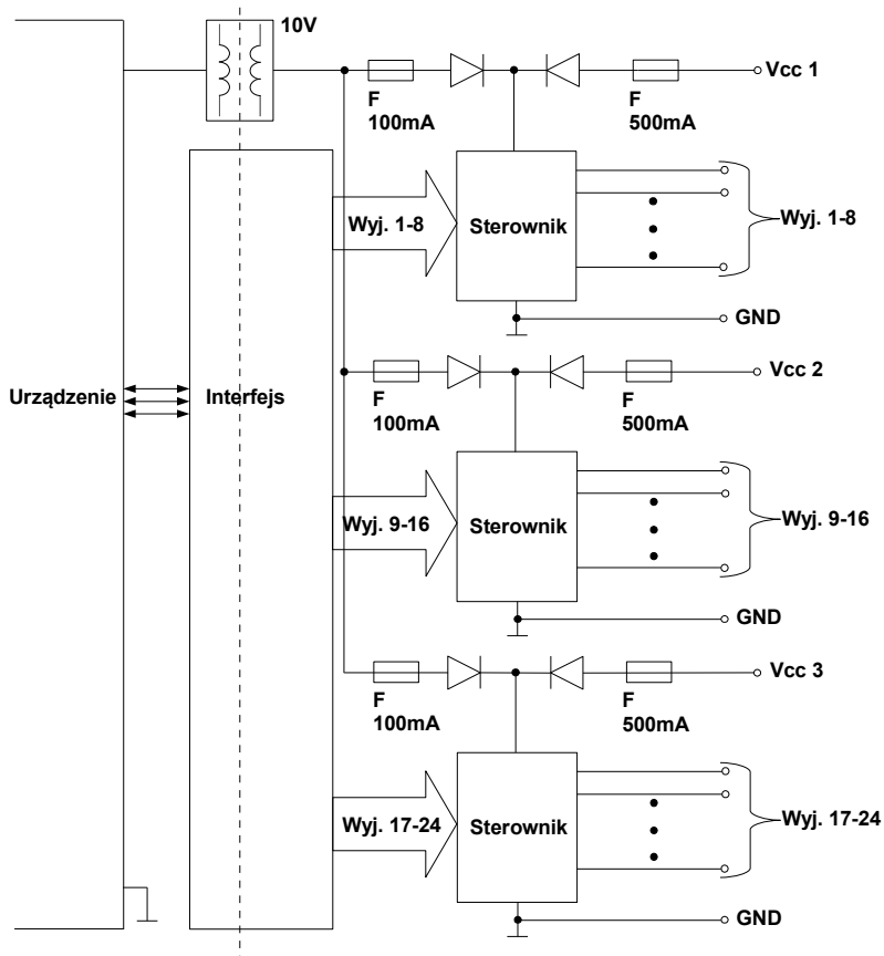
Rys. 8.26. Struktura wewnętrzna modułu wyjściowego SSR (24 wyjścia)
