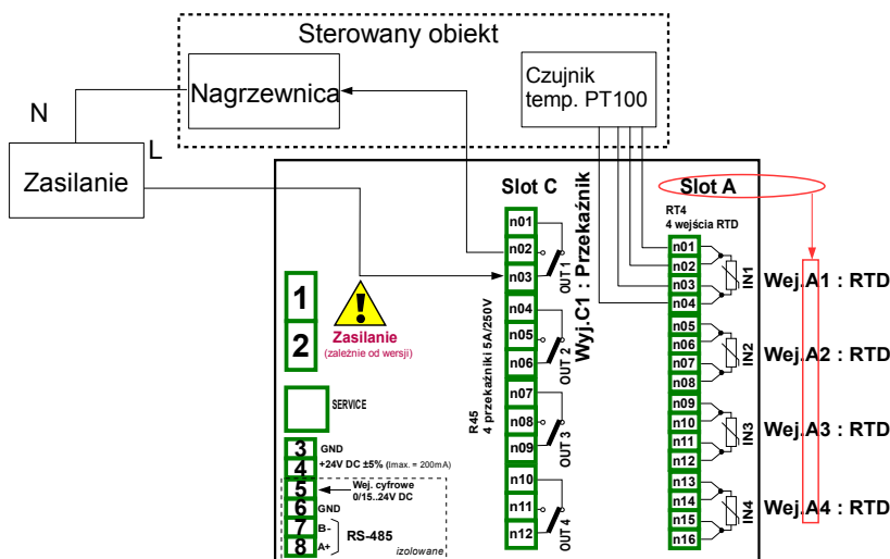
Rys. 7.96. Przykładowy sposób podłączenia do wejścia RTD i wyjścia przełącznikowego
