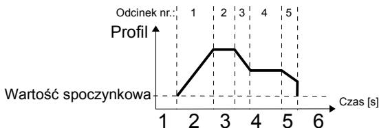
Rys.7.107. Przykładowy przebieg Profil/timera
