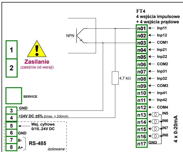
Rys. 8.12. Schemat połączeniowy dla modułu FT4 i czujnika typu NPN
