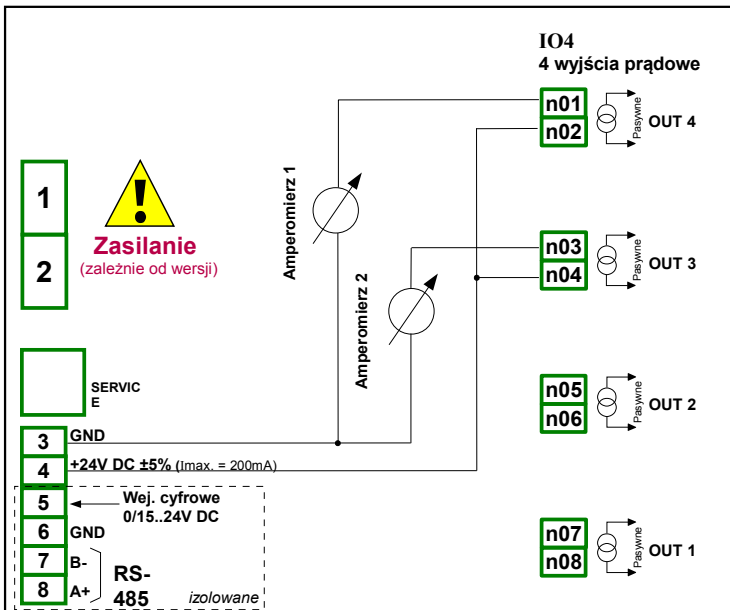
Rys. 8.31. Podłączenia dla Pasywnego wyjścia prądowego od strony zasilania
