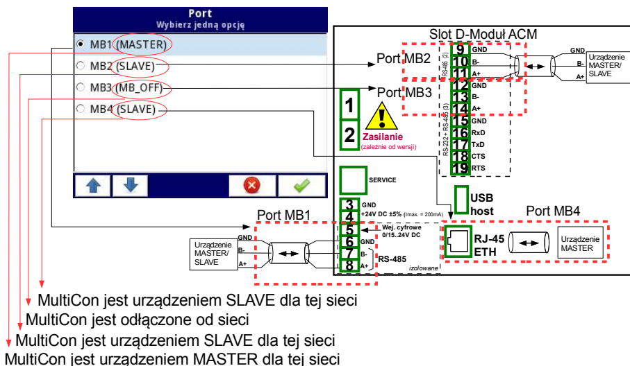
Rys. 7.51. Przykładowe podłączenie urządzenia MultiCon w sieci z podglądem skonfigurowanych portów Modbus
