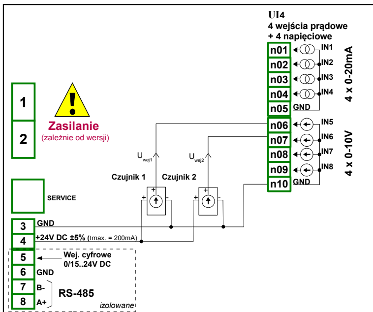
Rys. 8.6. Podłączenia przetworników napięciowych 3 przewodowych
