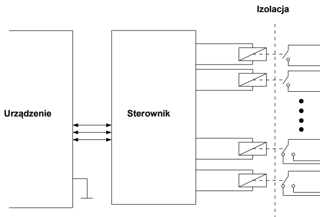
Rys. 8.28. Struktura wewnętrzna modułów wyjść przekaźnikowych
