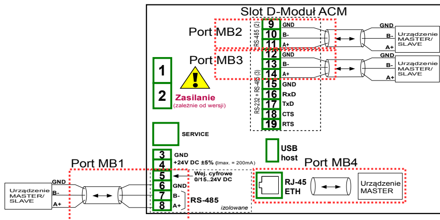
Rys. 7.135. Szeregowe porty komunikacyjne dostępne w urządzeniu
