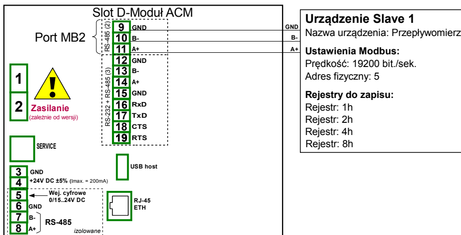
Rys. 7.140. Schemat połączeniowy dla portu modbusowego MB2
