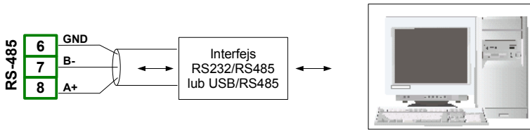
Rys. 4.23. Podłączenie sygnałów transmisji RS 485
