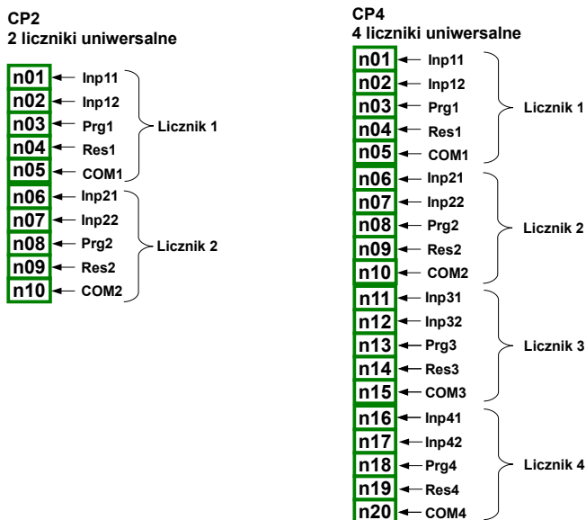
Rys. 8.19. Optoizolowane moduły liczników uniwersalnych
