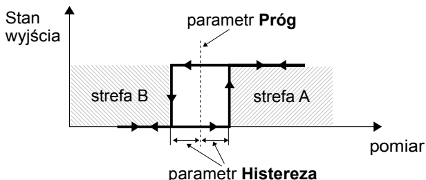
Rys. 7.85. Sterowanie jednoprogowe wyjścia przełącznikowego
