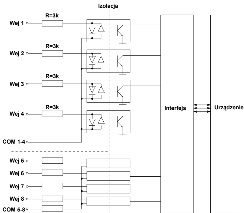
Rys. 8.18. Struktura wewnętrzna optoizolowanego modułu wejść cyfrowych
