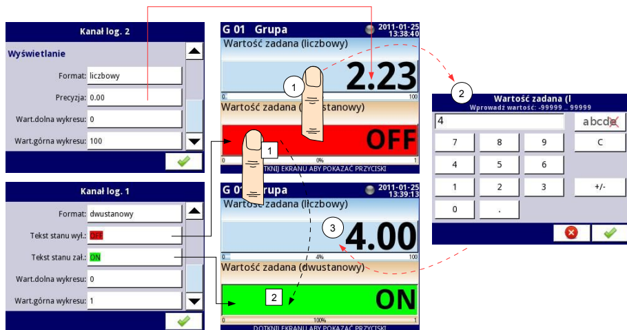
Rys. 7.55. Zasada działania przycisku dla formatu liczbowego i dwustanowego
