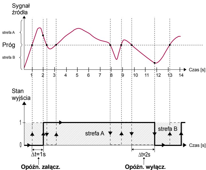
Rys. 7.88. Zasada pracy wyjść przekaźnikowych dla przykładowych ustawień czasowych: Opóźn.załącz. = 1 sec., Opóźn.wyłąc. = 2 sec.
