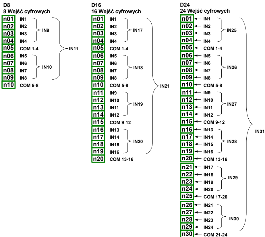
Rys. 8.17. Moduły wejść cyfrowych
