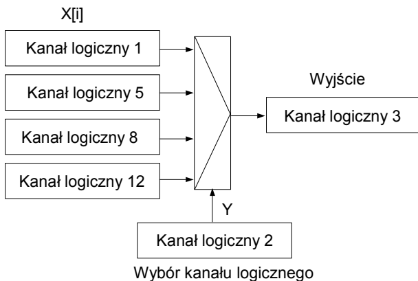
Rys. 7.75. Schemat blokowy działania funkcji matematycznej X[i] wybieranej przez Y
