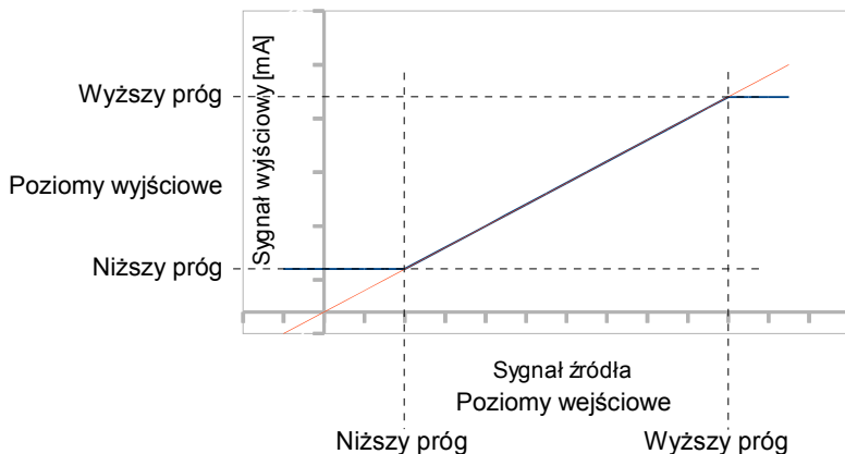
Rys. 7.94. Zależność sygnału wyjściowego (niebieski) od wejściowego (czwarty) dla Wyjścia prądowego
