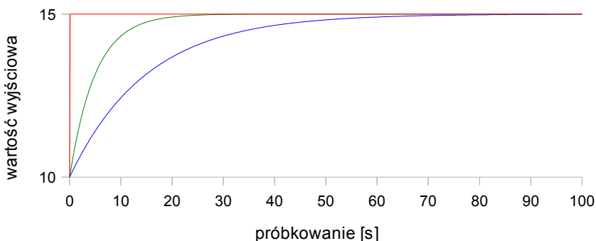
Rys. 7.40 Przykładowy przebieg sygnału wejściowego (wykres czerwony) oraz sygnał przefiltrowany dla w=5 (wykres zielony) i w=15 (wykres niebieski)
