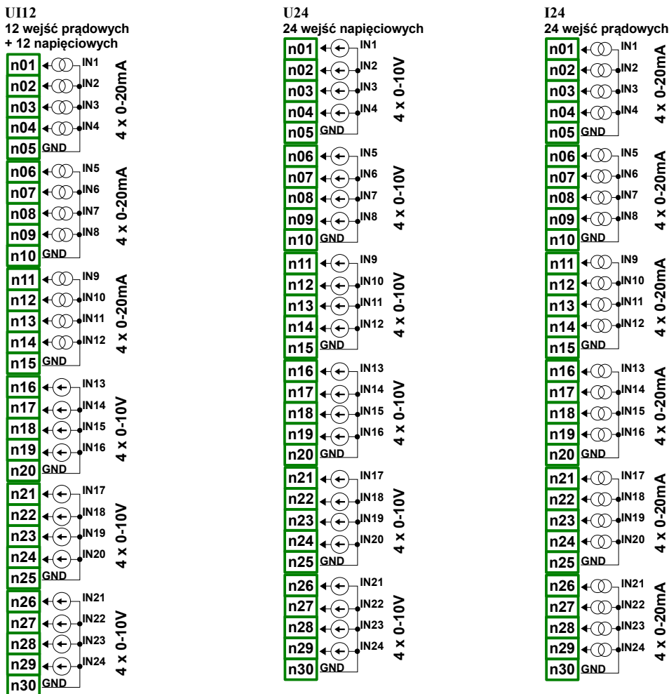
Rys. 8.3. Moduły napięciowe i prądowe cd.
