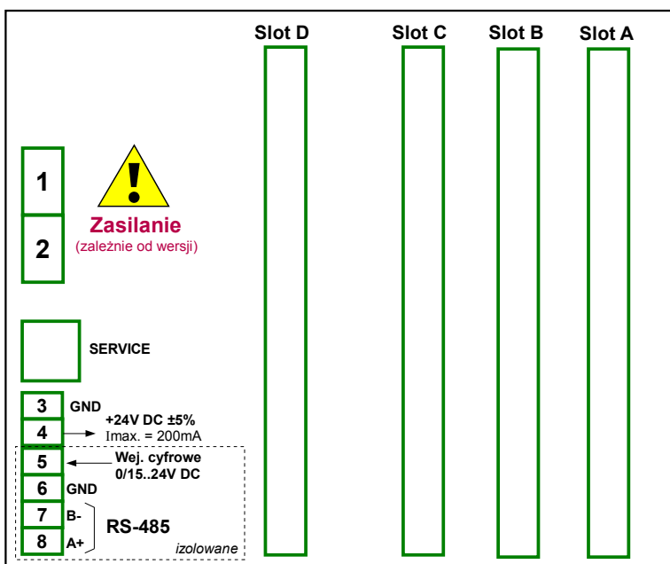
Rys. 4.8. Opis wyprowadzeń
