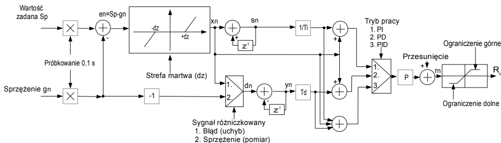
Rys. 7.115. Schemat blokowy Regulatora zaimplementowanego w urządzeniu
