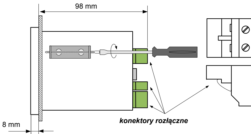
Rys. 4.4. Mocowanie za pomocą uchwyty
