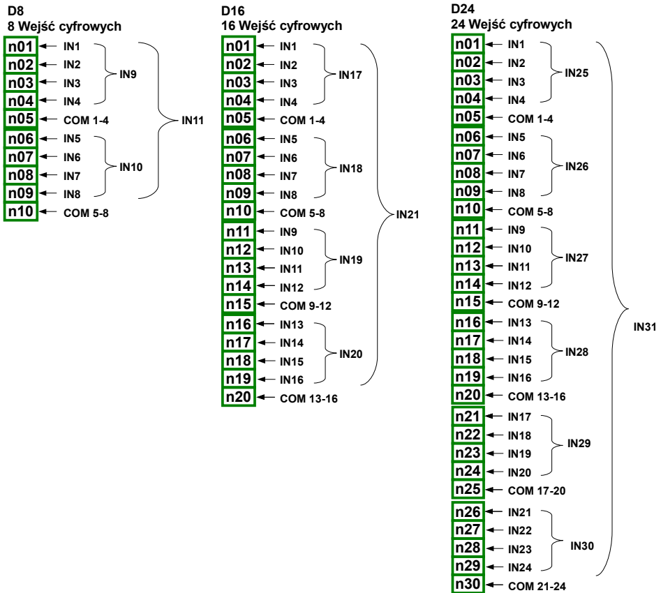
Rys. 4.17. Moduły wejść cyfrowych
