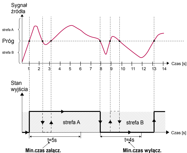
Rys. 7.89. Zasada pracy wyjść przekaźnikowych dla przykładowych ustawień czasowych: Min.czas załącz. = 5 sec., Min.czas wyłąc. = 4 sec.
