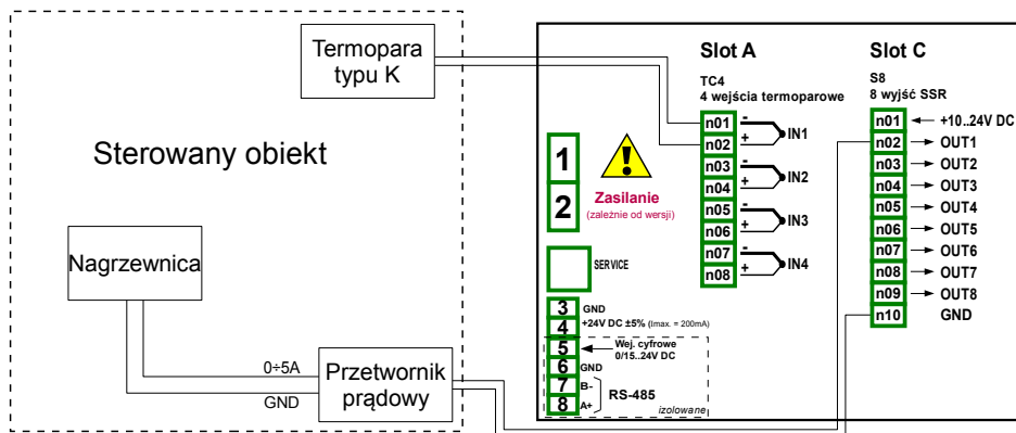
Rys. 7.117. Schemat połączeniowy dla modułów TC4 oraz S8
