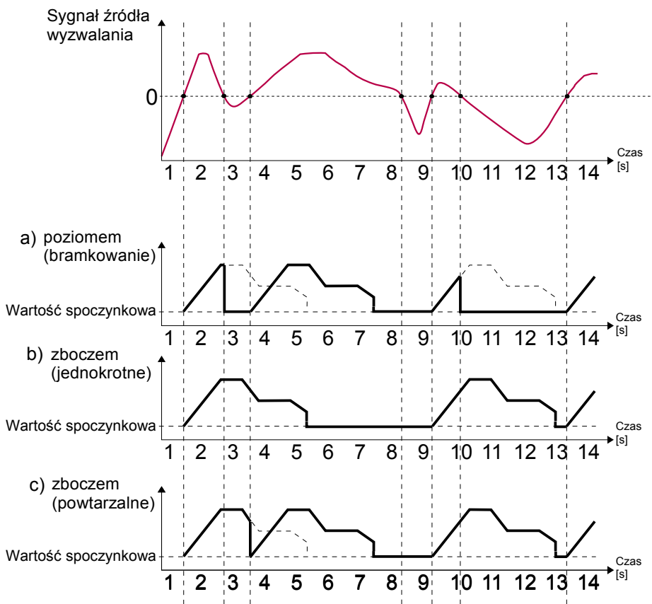
Rys.7.108. Przykładowe przebiegi wyjściowe Profilu zdefiniowanego na Rys.7.107 wyzwalanego sygnałem źródła wyzwalania dla Trybu wyzwalania: poziomem (bramkowanie), zбочem (jednokrotne), zбочem (powtarzalne)
