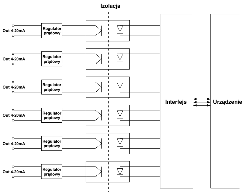
Rys. 8.32. Struktura wewnętrzna modułów wyjść prądowych
