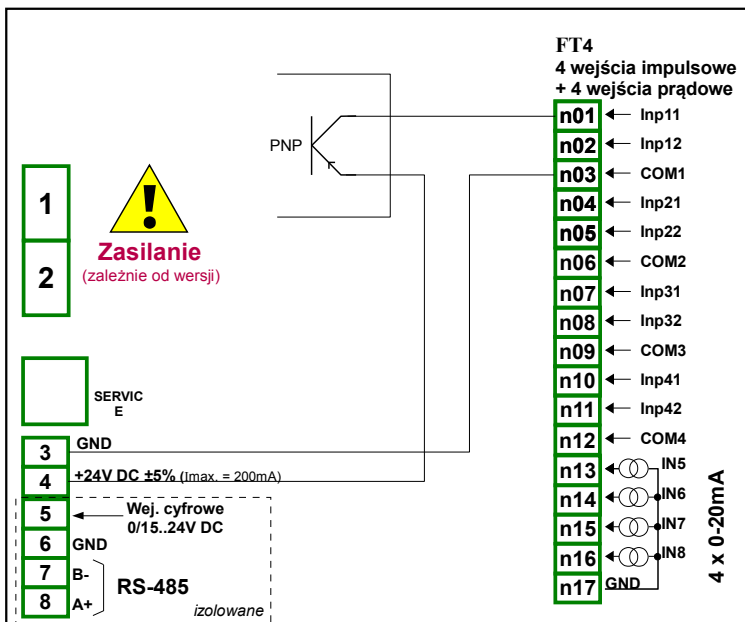
Rys. 7.78. Schemat podłączeniowy modułu FT4 i czujnika typu PNP
