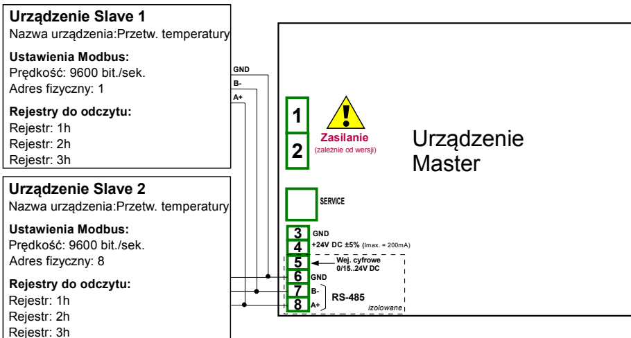
Rys. 7.73. Schemat połączeniowy dla portu modbusowego MB1
