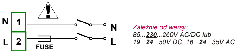
Rys. 4.6. Podłączenie zasilania
