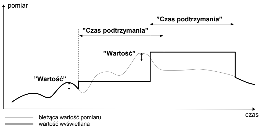
Rys. 7.41. Sposób detekcji wartości szczytowych
