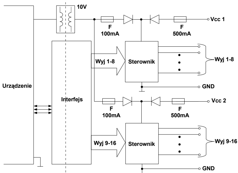
Rys. 8.25. Struktura wewnętrzna modułu wyjściowego SSR (16 wyjść)
